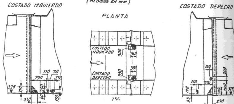
FIGURA 6 COMPUERTA DE SERVICIO (MEDIDAS EN MM)
